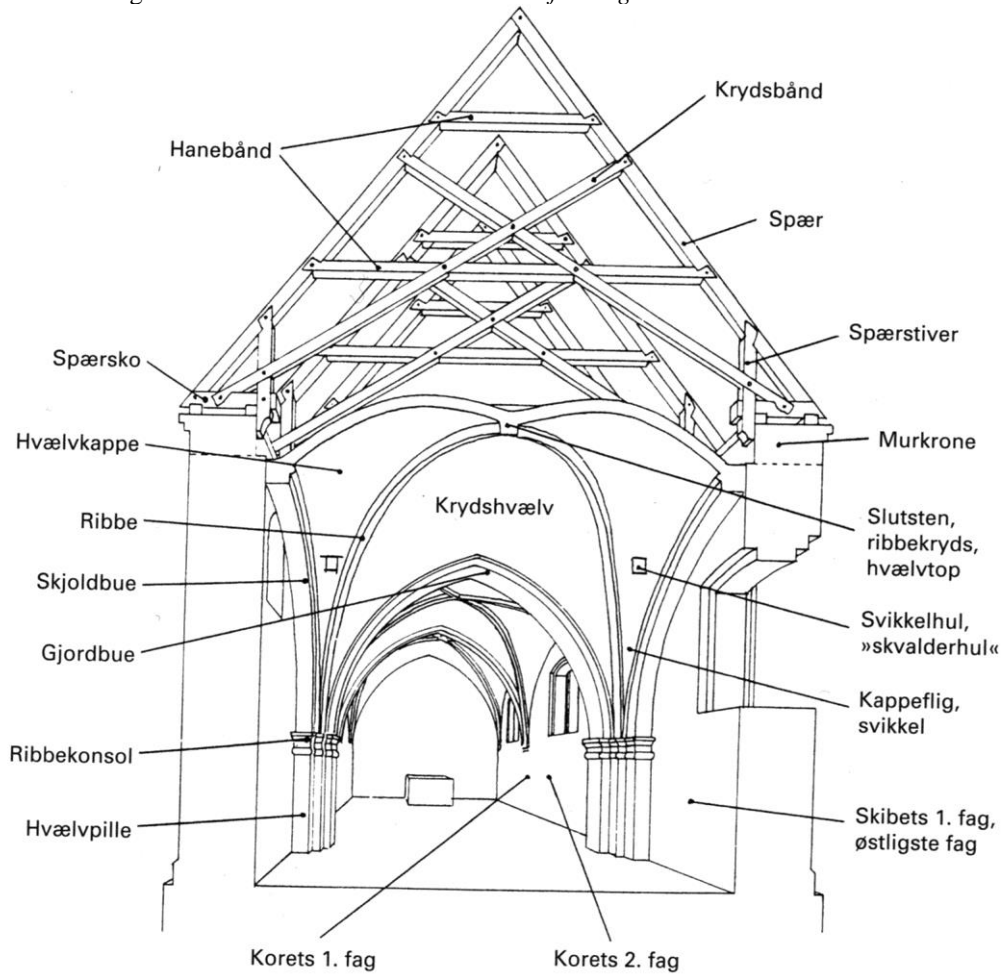
Figur 6: Det gotiske landsbykirkerum (kor og skib) med hvælvinger, vinduer, ribber og højalter.
