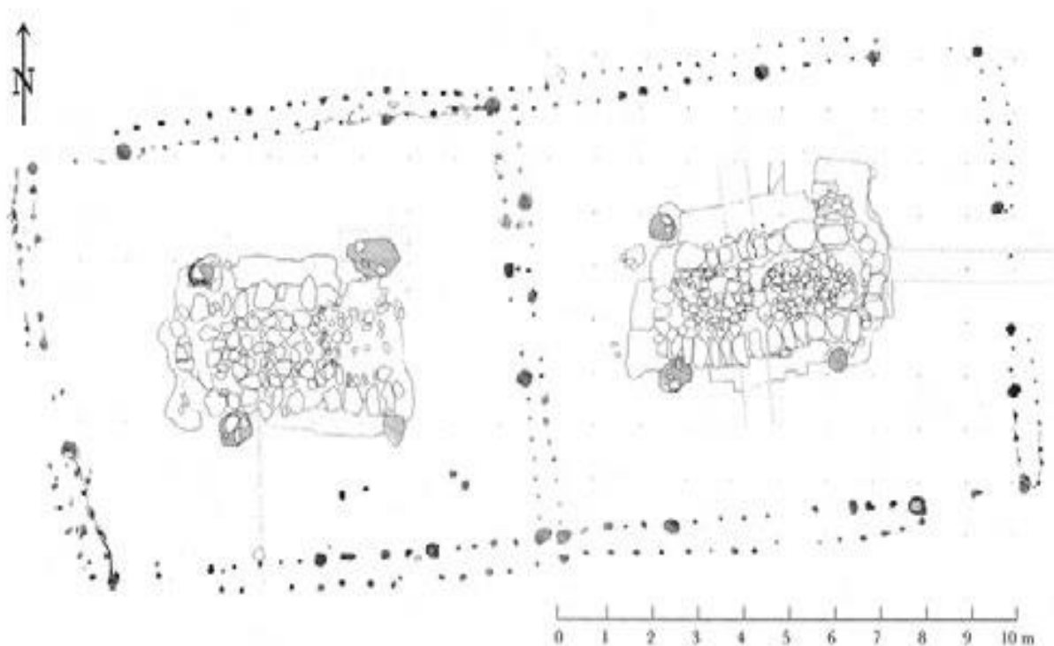
KORT 4: En udgravet 'dobbeltthytte', der nu er rekonstrueret på Læsø Saltsyderi. De to sydehytter består inderst af et ildsted opbygget af kampesten og græstørv. Taget og de to sydepander har hver været holdt oppe af 4 stolper af svært tømmer. Ydervæggene bestod af to lag flettede grene mellem lodrette rafter. Man har fyldt væggene med ålegræs op til ca. 1–1½ m højde, for at beskytte ildstedet ved højvande og mod blæsevejr. Kilde: Hans Langballe, J. Velle, Hikuin 1993.
